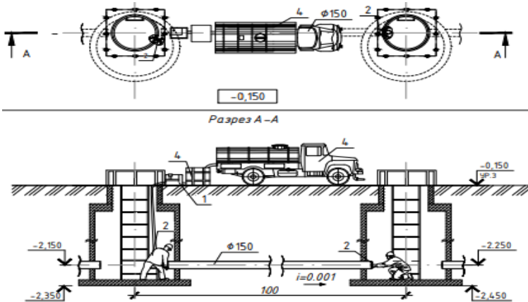
Рис. 7. Дезинфекция трубопровода.
