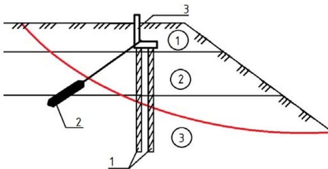
Рис. 9. Схема усиления оползневого склона с помощью свай ЭРТ и грунтобетона: 1 – сваи ЭРТ; 2 – грунтобетонный анкер; 3 – угловая монолитная ж/б подпорная стена; (1)–(3) – инженерно-геологические элементы
