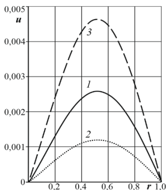
Рис. 4. Изменение радиального перемещения вдоль радиуса пластины
