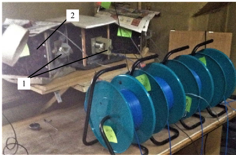
Рис. 1. Внешний вид части экспериментального оборудования. На рисунке показано магнитные прижимы с закрепленными преобразователями АЭ (1), опалубка с бетонной смесью внутри (2)
