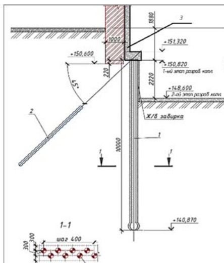
Рис. 4. Шпунтовая стена ограждения котлована из буроинъекционных свай и грунтовых анкеров ЭРТ:
