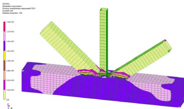
Рис. 5. Изополя эквивалентных напряжений в узле фермы
