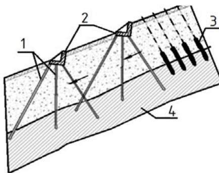
Рис. 8. Противооползневая защита склонов из буроинъекционных свай ЭРТ и нагелей (шпонок): 1 – сваи в составе подпорной сетчатой стены; 2 – уголковая сетчатая подпорная стена; 3 – нагели (шпонки) в плоскости сдвига; 4 – плоскость сдвига
