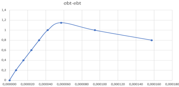
Рис. 3. Диаграмма участка растяжения для бетона В30
