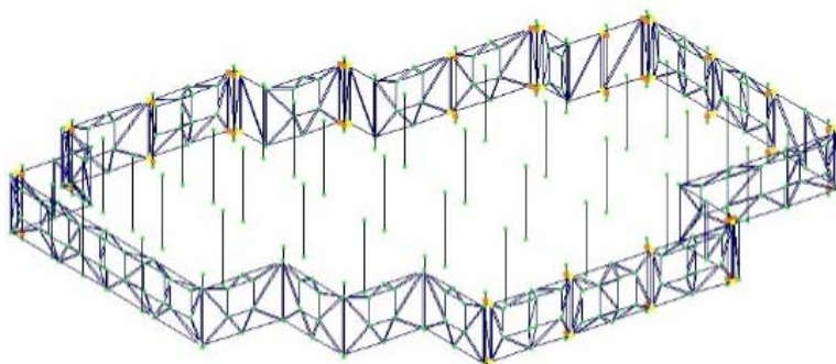
Рис. 11. Собранная модель этажа здания для дальнейшей работы и анализа нагрузок в ПК Лира-САПР
