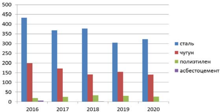
Рис. 2. Ликвидация повреждений трубопроводов систем водоснабжения по видам материалов, шт.
