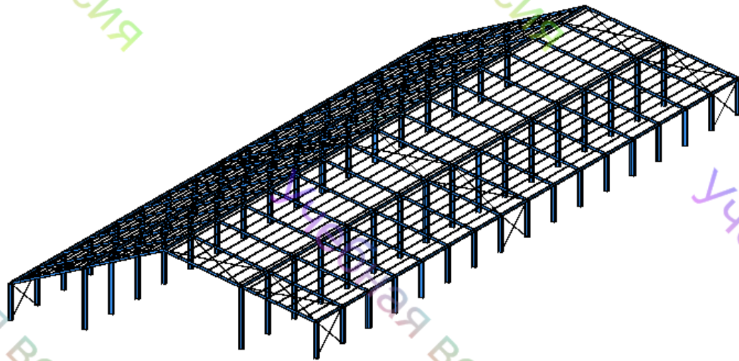
Рис. 1 Пространственная модель
