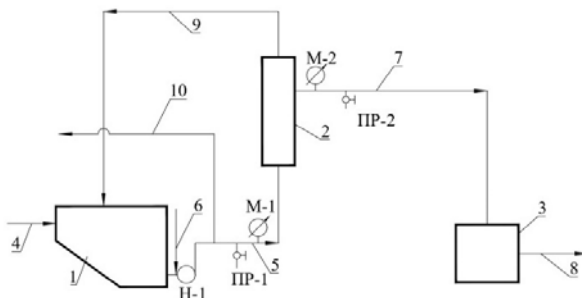
Рисунок 1 – Технологическая схема экспериментальной установки
