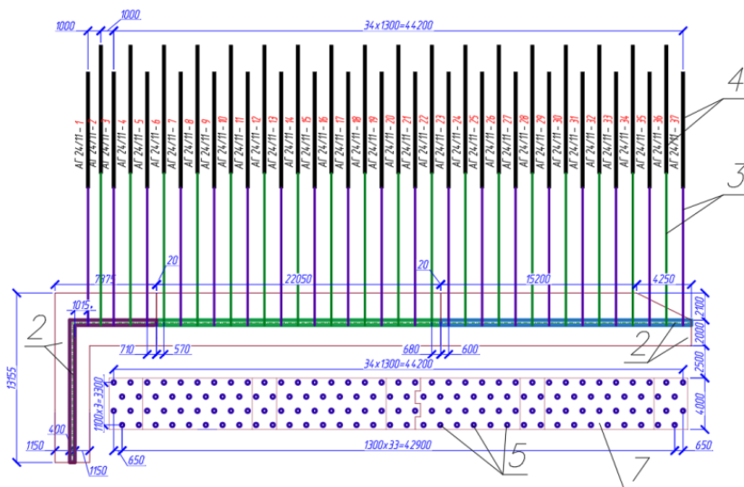
Рисунок 1 – Схема устройства монолитных железобетонных ростверков и диафрагм на завершающем этапе:
