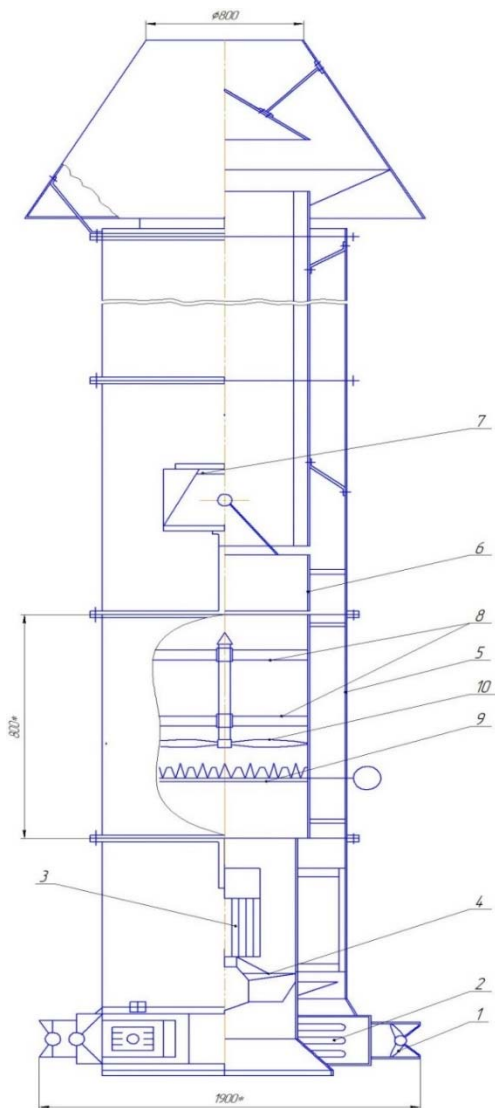
Рисунок 1 – Модернизированная приточно-вытяжная установка.
